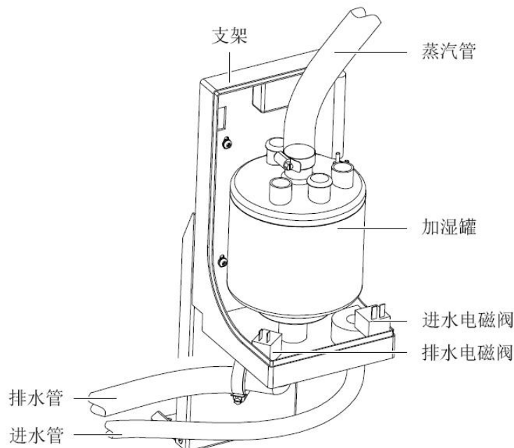
图 6.2.5 电极加湿器示意图
