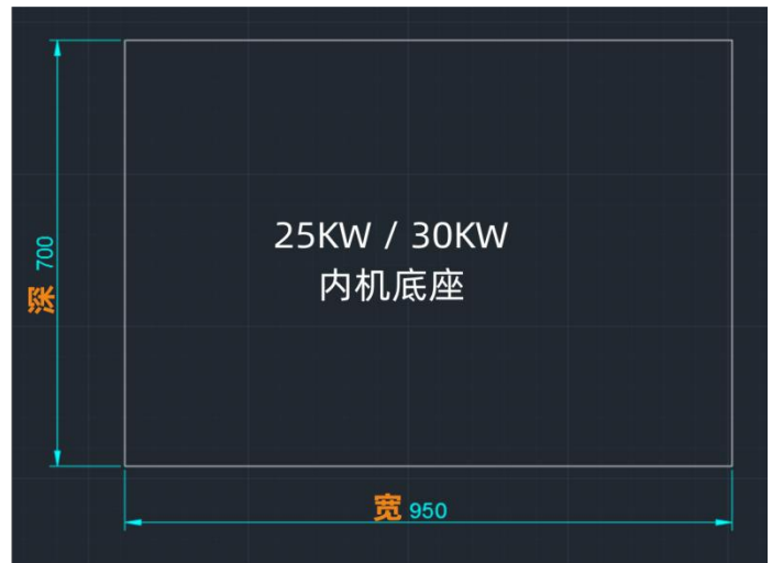
25KW / 30KW 内机底座规格
