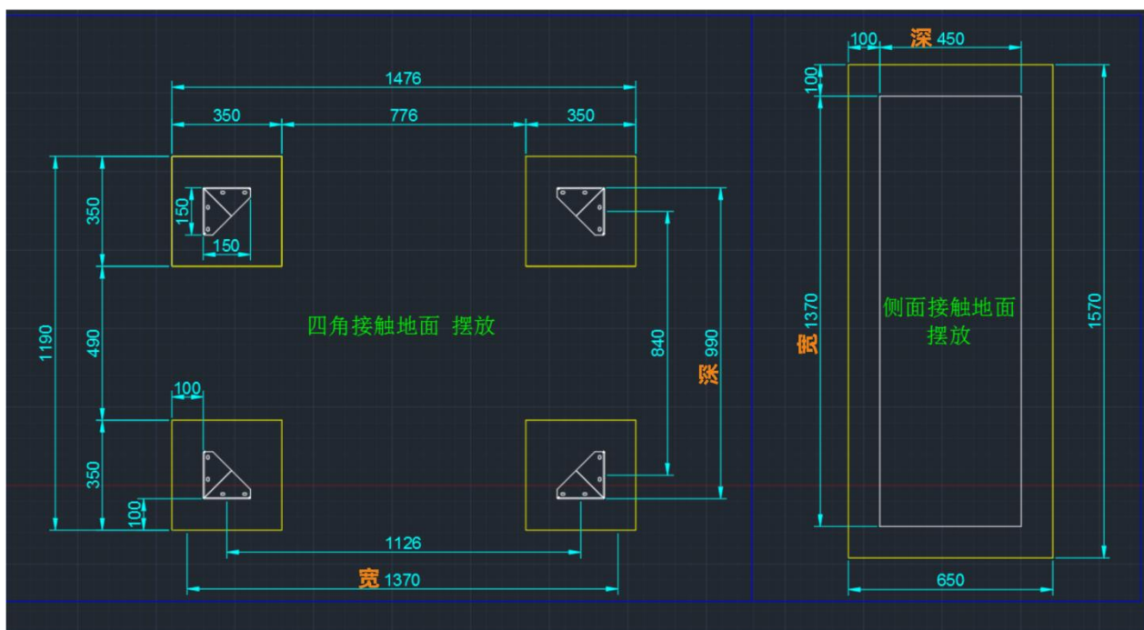
30KW 外机底座规格
