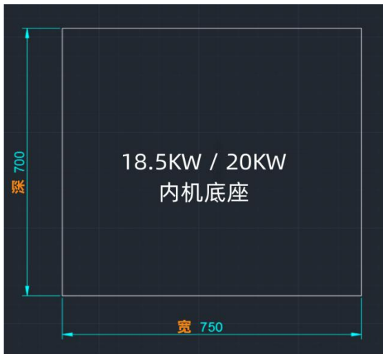
18.5KW / 20KW 内机底座规格
