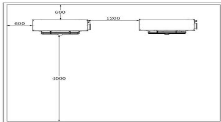
图 2.5.1.1 室外机竖直安装示意图（单位：mm）
