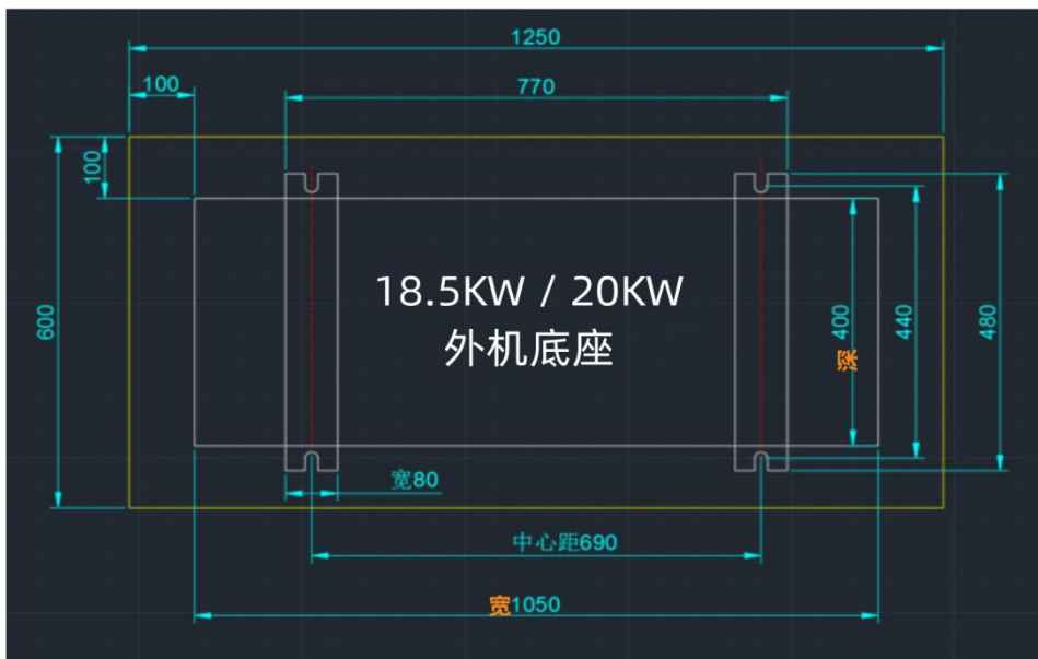
18.5KW / 20KW 外机底座规格
