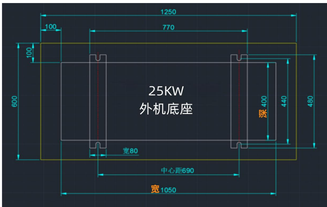
25KW 外机底座规格
