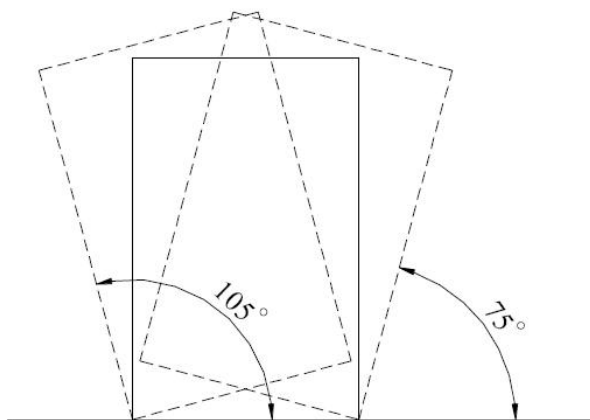
图 2.1.2 搬运倾角
