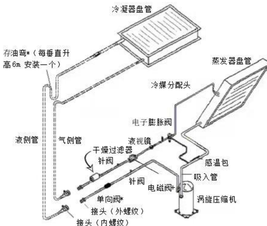
图 2.3.1 空调总体布局图
